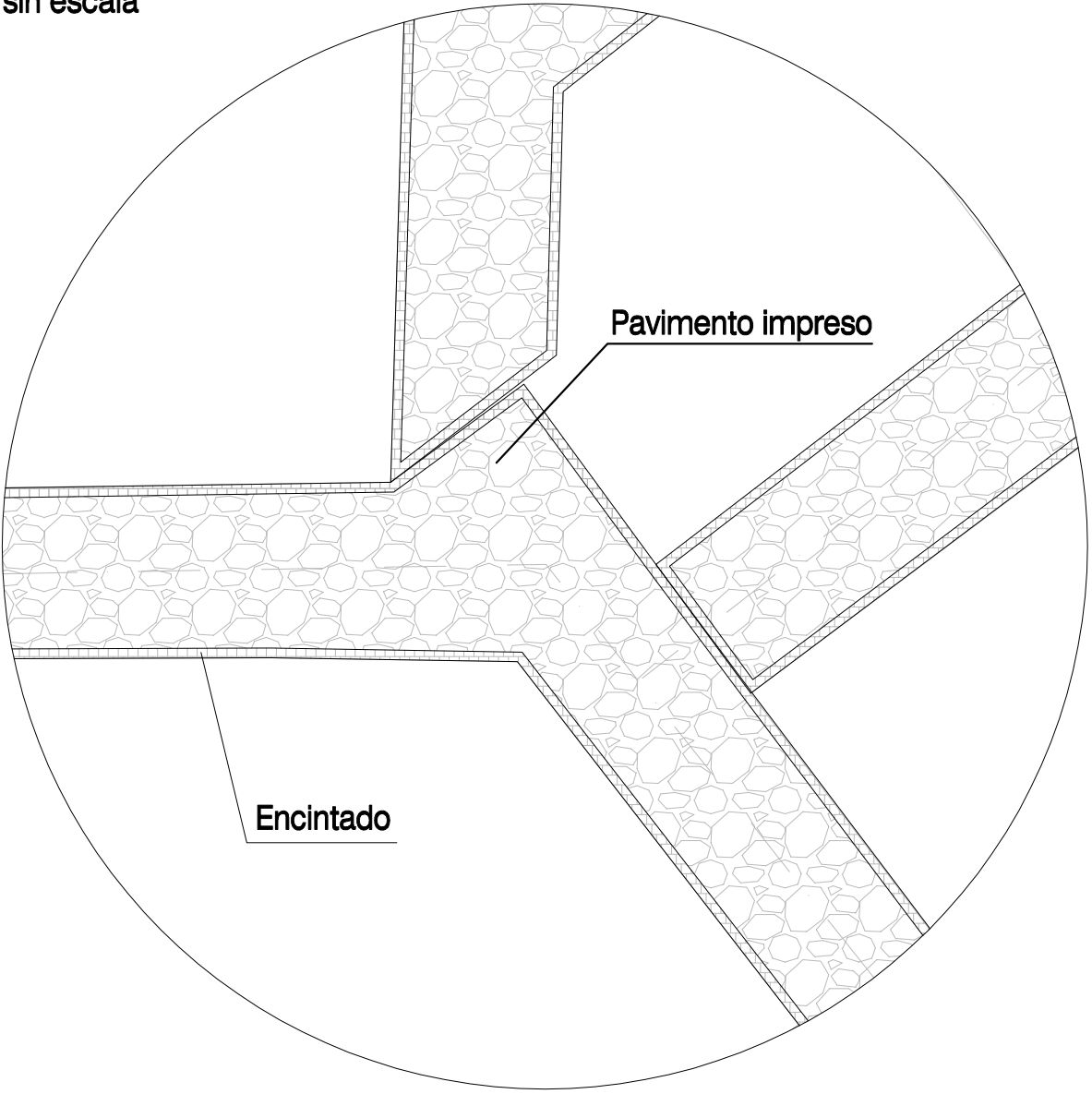
DETALLE PAVIMENTO sin escala
