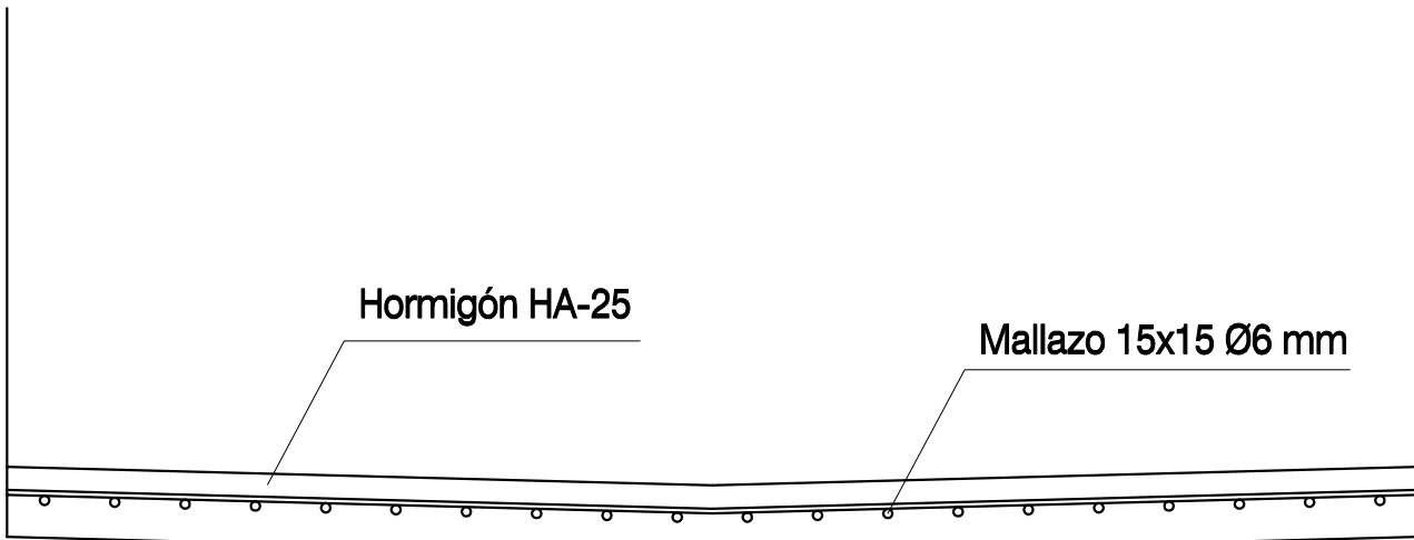
SECCIÓN CALZADA TIPO: Pendiente central sin escala
