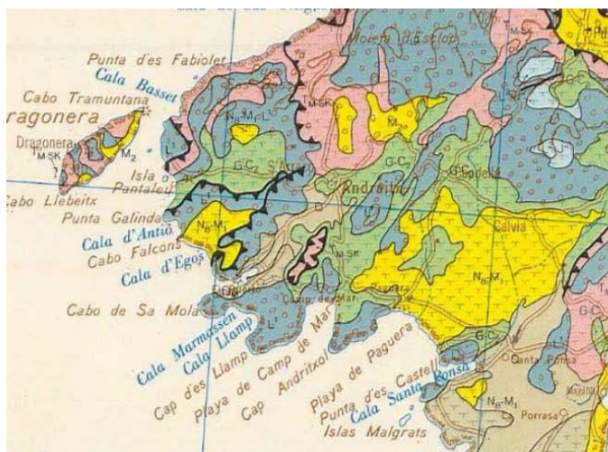
(dominis geomorfològics de la zona de Andratx)
